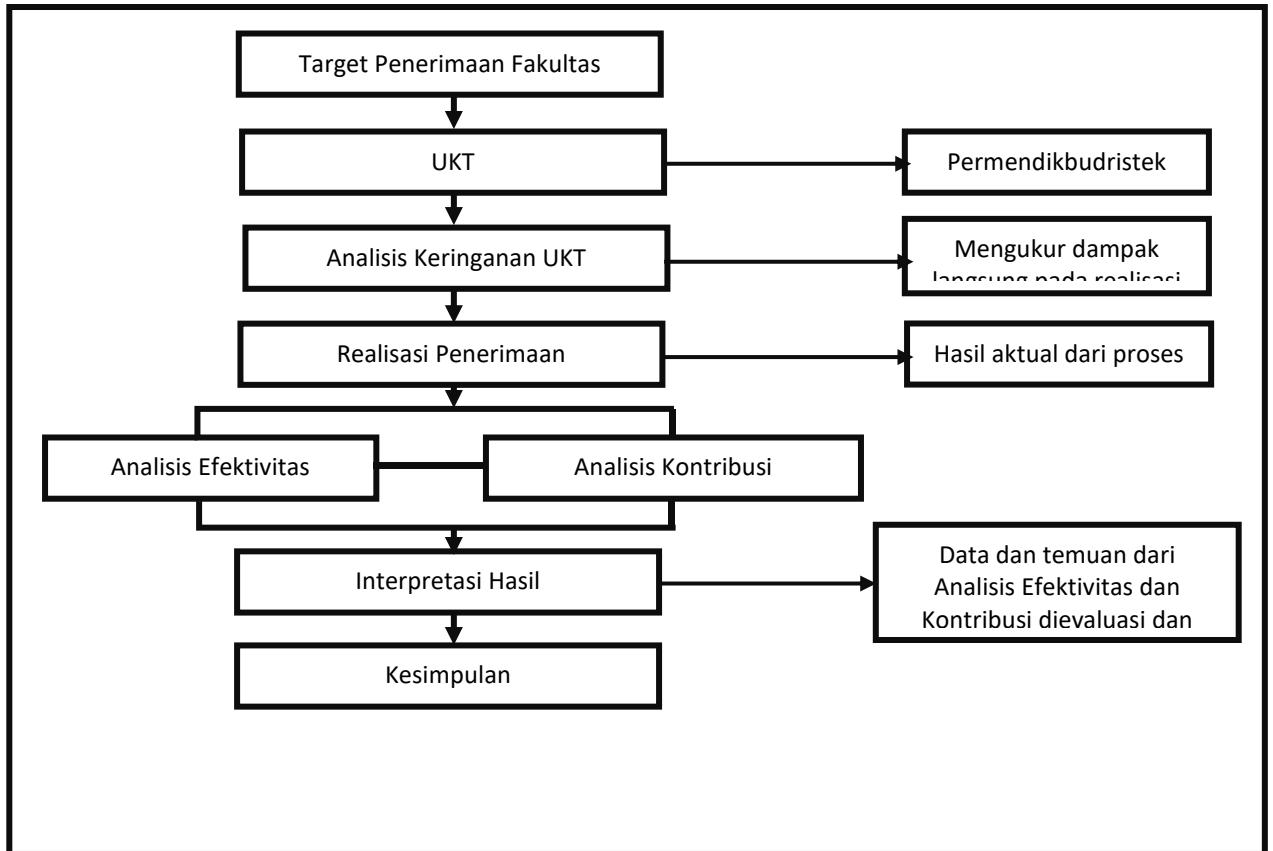
Gambar 2.1 Alur Pemikiran
