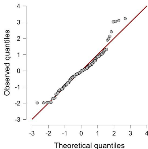
Gambar 2 Uji Normalitas
