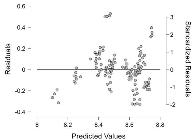
Gambar 3 Uji Homogenitas
